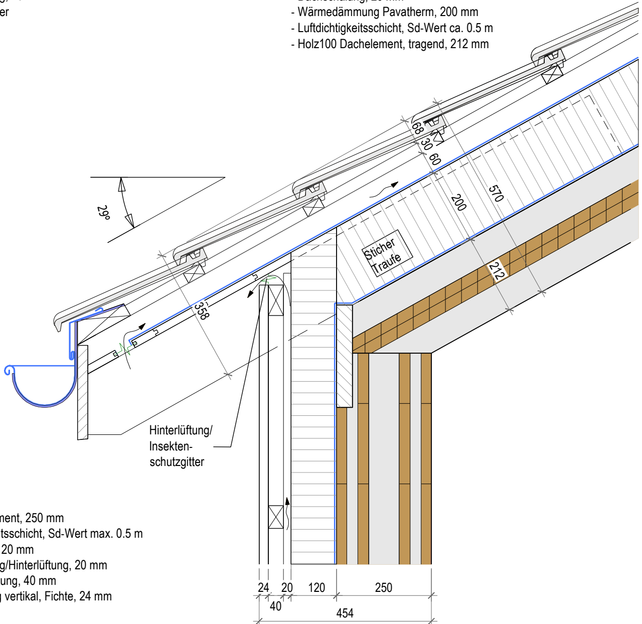
Vertikalschnitt 1:10
